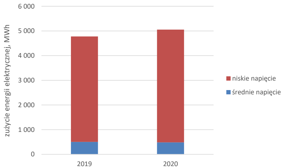
Rysunek 11 Zużycie energii elektrycznej na terenie gminy Ślemień w latach 2019 – 2020
