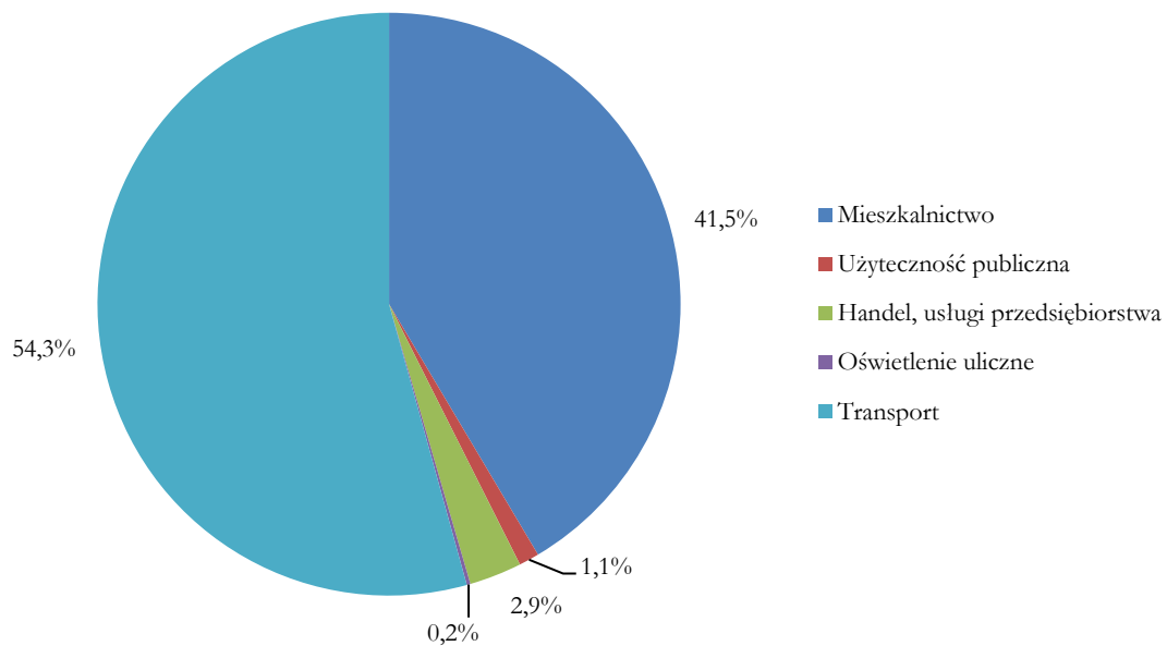
Rysunek 29 Struktura zużycia energii wg sektorów – ujęcie graficzne (rok kontrolny)
