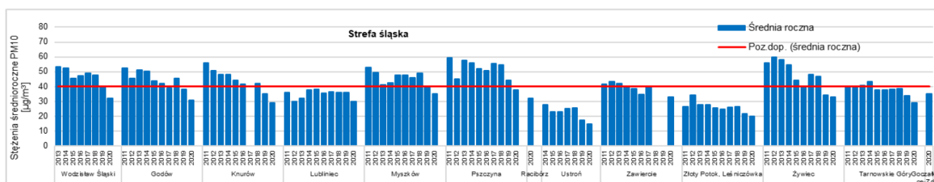
Rysunek 20 Przebieg wartości średniorocznej stężenia pyłu PM 10 na poszczególnych stanowiskach pomiarowych w województwie śląskim w strefie śląskiej na tle poziomu dopuszczalnego w latach 2011 – 2020 źródło: Roczna ocena jakości powietrza w województwie śląskim. Raport wojewódzki za rok 2020.
