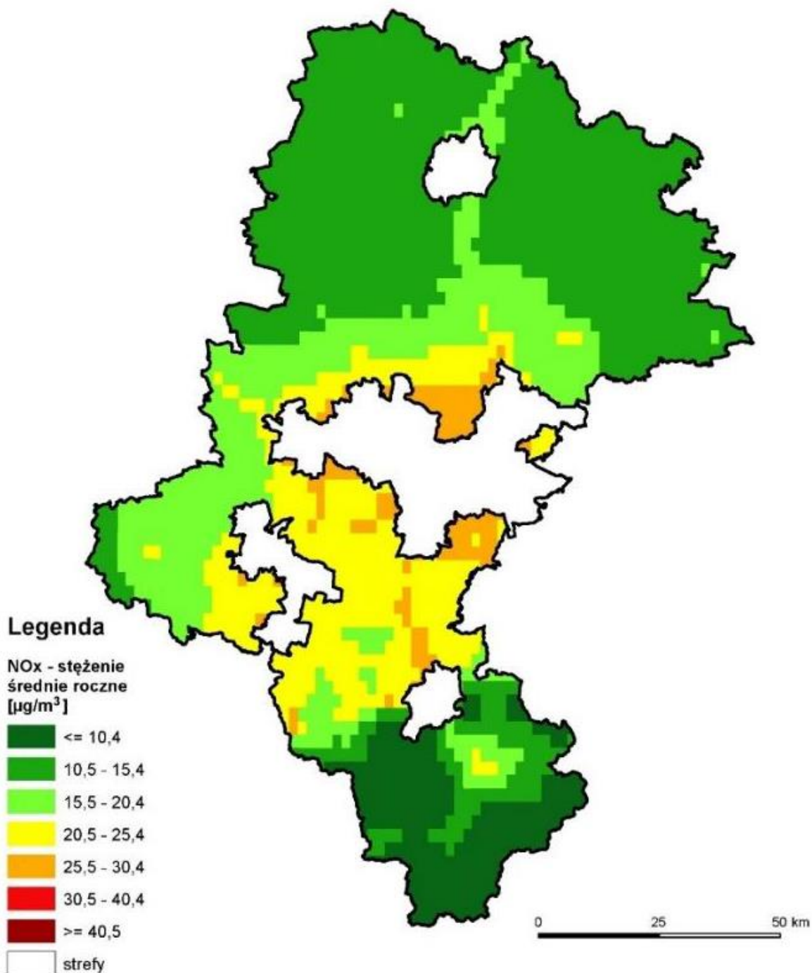
Rysunek 17 Rozkład przestrzenny wartości stężenia średniorocznego tlenków azotu w województwie śląskim w 2020 roku, opracowany z wykorzystaniem metody szacowania w oparciu o wyniki modelowania jakości powietrza dla roku 2020 wykonanego przez IOŚ-PIB
