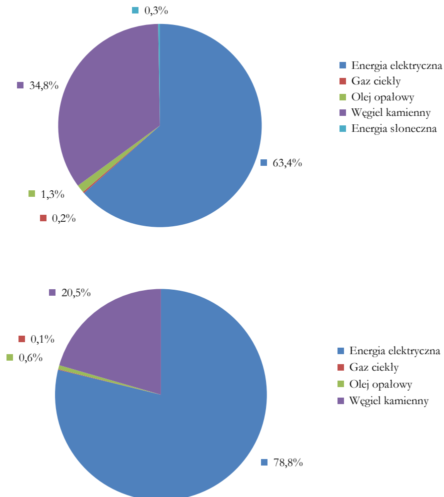
Rysunek 25 Struktura zużycia energii oraz emisji CO 2 – obiekty: handel, przemysł, usługi (rok kontrolny)
