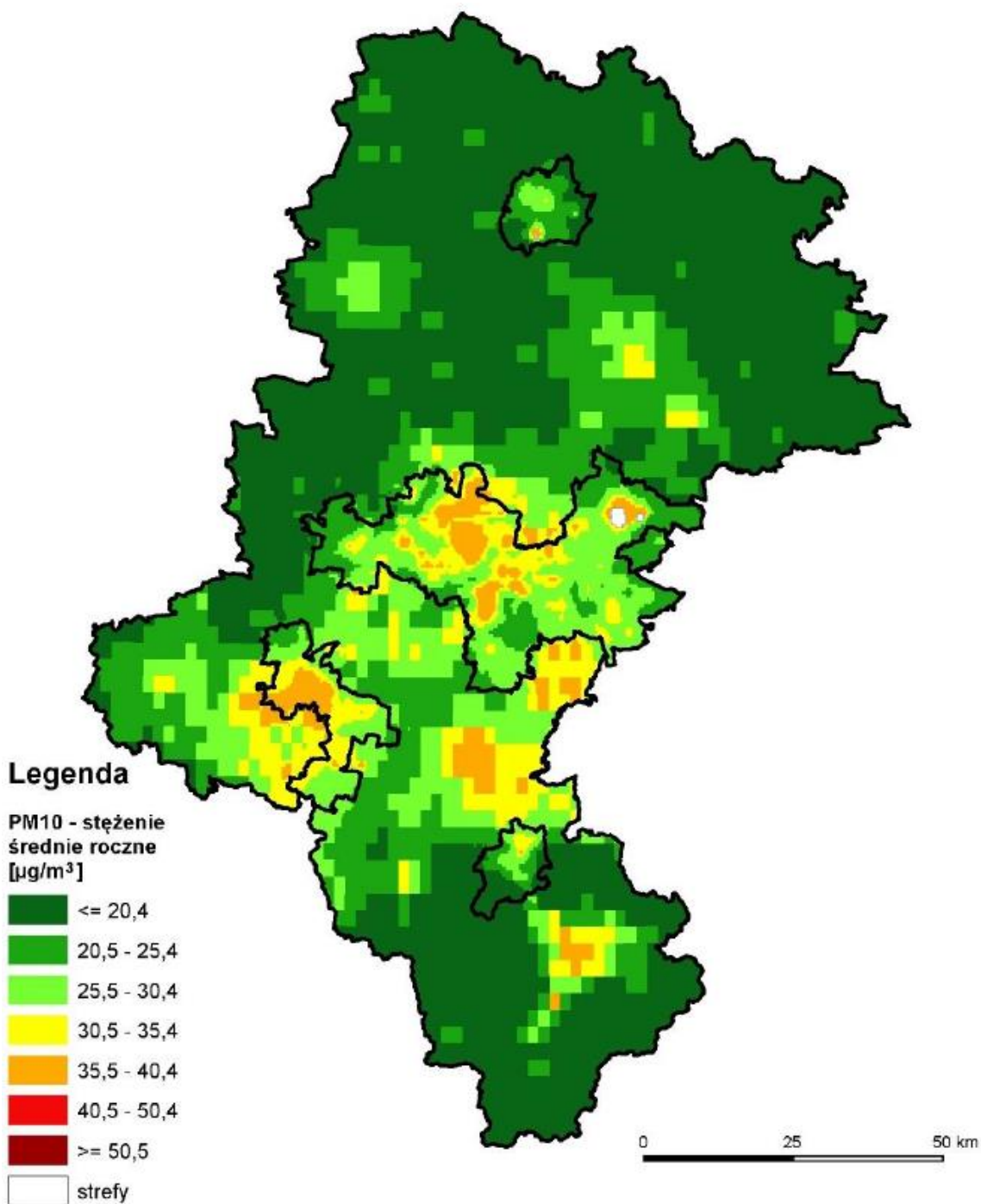
Rysunek 13 Rozkład przestrzenny wartości stężenia średniorocznego pyłu PM10 w województwie śląskim w 2020 roku, opracowany z wykorzystaniem metody szacowania w oparciu o wyniki modelowania jakości powietrza dla roku 2020 wykonanego przez IOŚ-PIB
