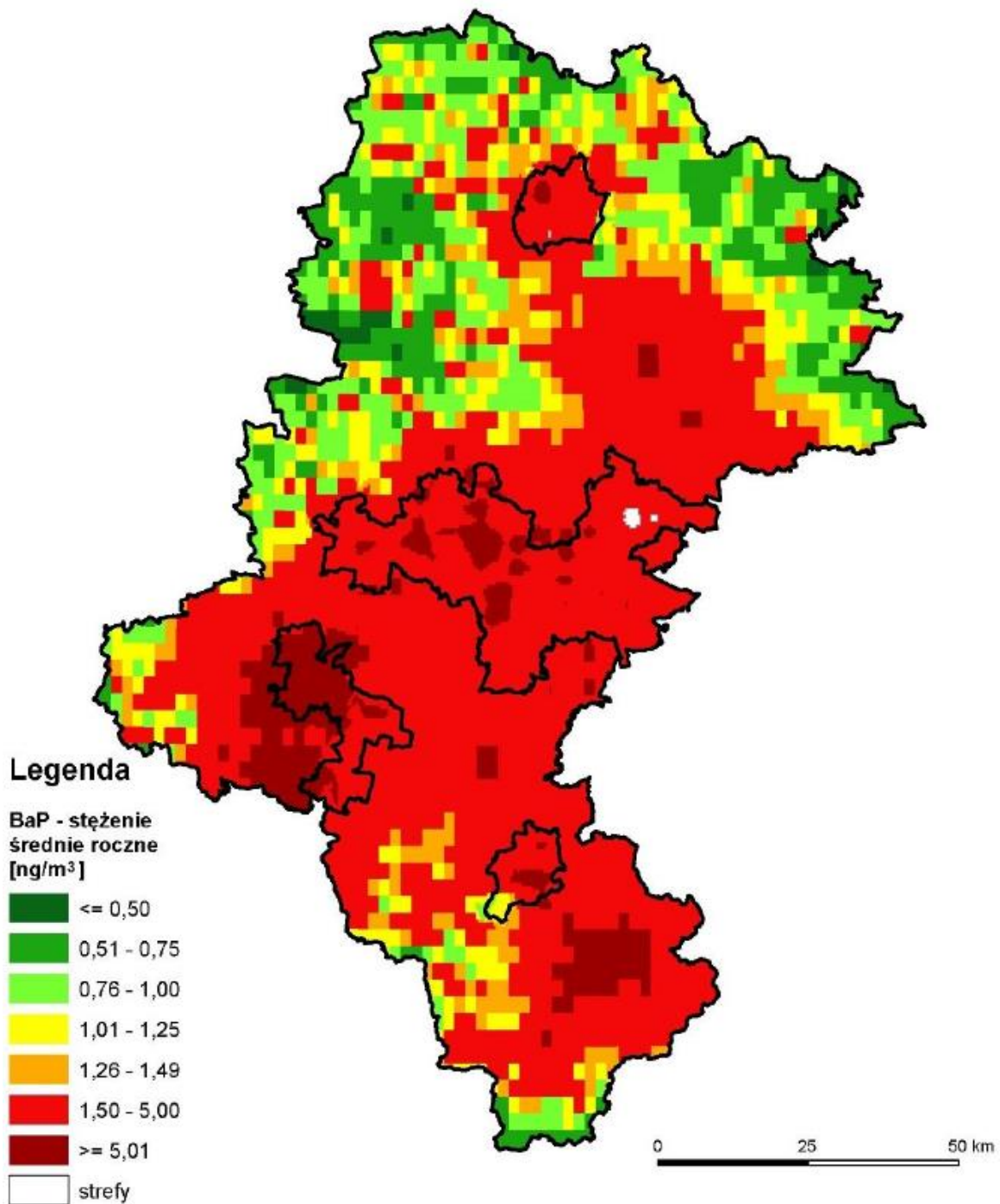
Rysunek 15 Rozkład przestrzenny wartości stężenia średniorocznego benzo(a)pirenu w pyłe PM10 w województwie śląskim w 2020 roku, opracowany z wykorzystaniem metody szacowania w oparciu o wyniki modelowania jakości powietrza dla roku 2020 wykonanego przez IOŚ-PIB
