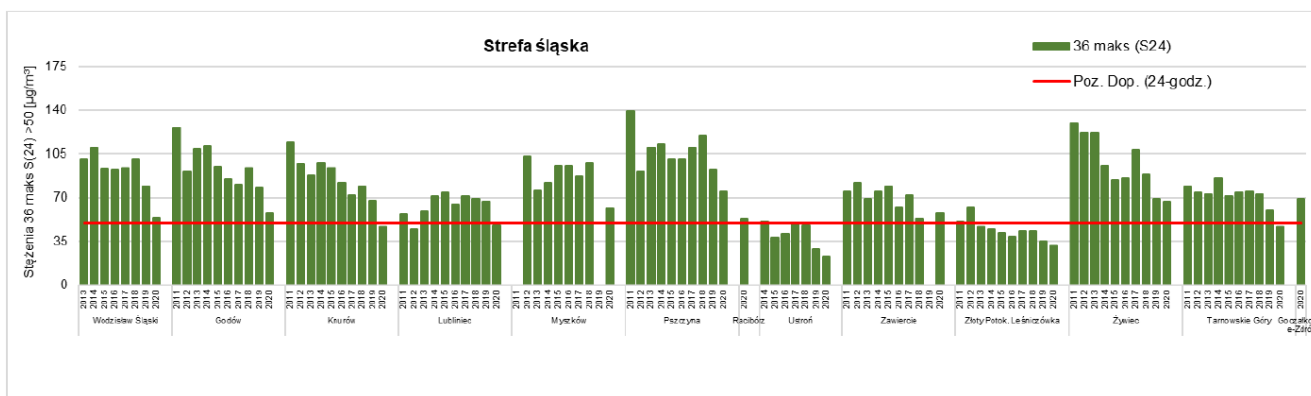
Rysunek 19 Przebieg 36 maksymalnej wartości 24-godzinowej stężenia pyłu PM 10 na poszczególnych stanowiskach pomiarowych w województwie śląskim w strefie śląskiej na tle poziomu dopuszczalnego w latach 2011 – 2020 źródło: Roczna ocena jakości powietrza w województwie śląskim. Raport wojewódzki za rok 2020.
