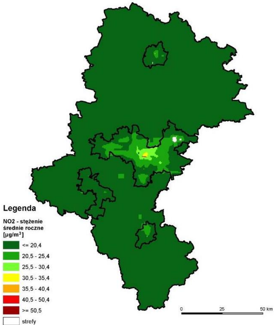
Rysunek 12 Rozkład przestrzenny wartości stężenia średniorocznego NO 2 w województwie śląskim w 2020 roku, opracowany z wykorzystaniem metody szacowania w oparciu o wyniki modelowania jakości powietrza dla roku 2020 wykonanego przez IOŚ-PIB
