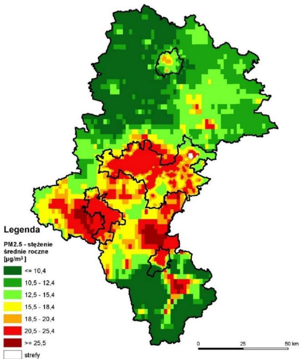
Rysunek 14 Rozkład przestrzenny wartości stężenia średniorocznego pyłu PM 2,5 w województwie śląskim w 2020 roku, opracowany z wykorzystaniem metody szacowania w oparciu o wyniki modelowania jakości powietrza dla roku 2020 wykonanego przez IOŚ-PIB
