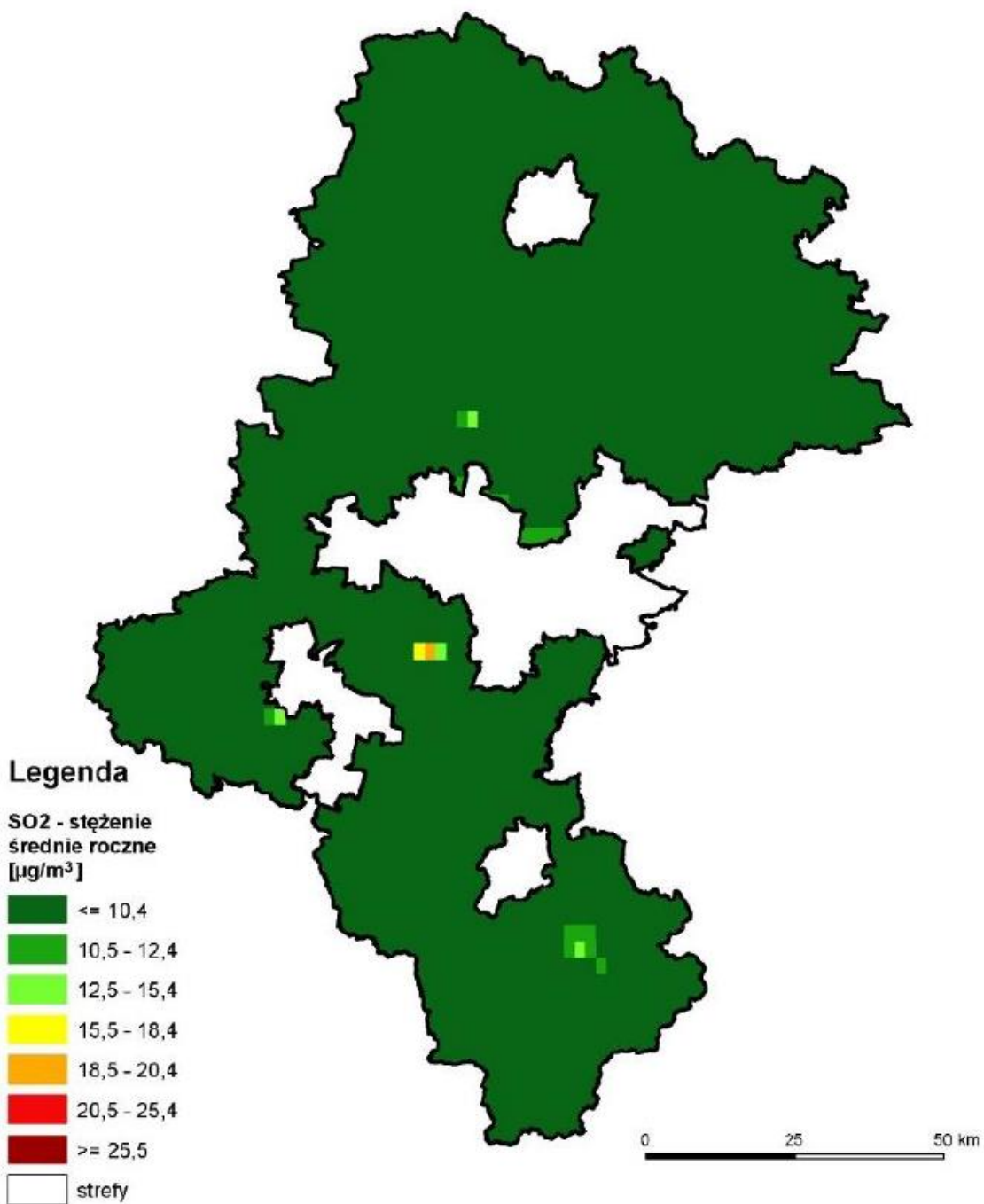
Rysunek 16 Rozkład przestrzenny wartości stężenia średniorocznego dwutlenku siarki w województwie śląskim w 2020 roku, opracowany z wykorzystaniem metody szacowania w oparciu o wyniki modelowania jakości powietrza dla roku 2020 wykonanego przez IOŚ-PIB
